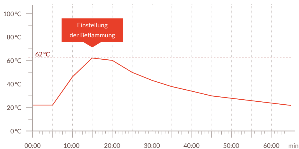
Darstellung der Temperaturkurve des untersten Thermoelements
