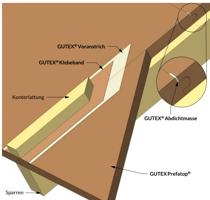
Stoßdetail/-abdichtung bei Dachelementen mit GUTEX Prefatop® (Detail 1.1.601)
